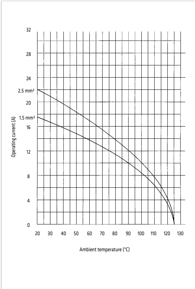
GW-ESHV RANGE 10P + 2P + \frac{1}{2} / 20P + 4P + \frac{1}{2}
